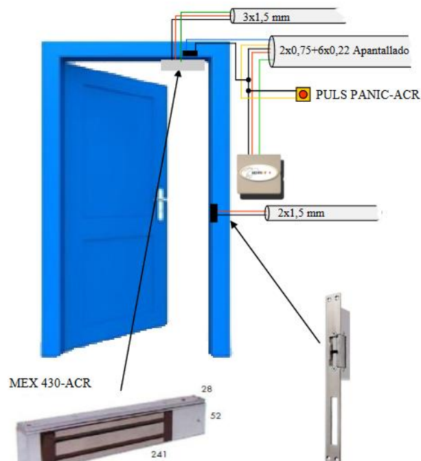
Esquema de les connexions per a una instal·lació de control d'accés a una porta estàndard
